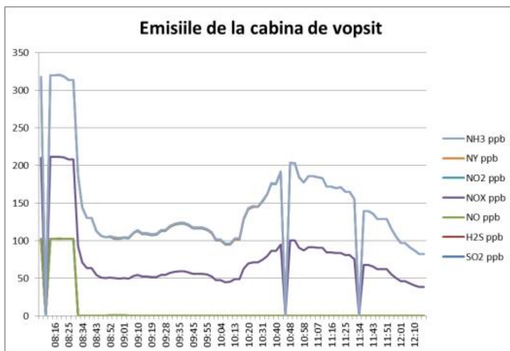
Figura 4 La ora 12:15 a fost oprită monitorizarea la cabina de vopsire deoarece nu mai existau repere pentru vopsit în ziua respectivă.
